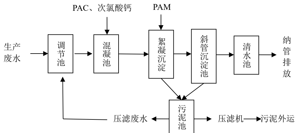
图 7-1 废水处理工艺流程示意图
